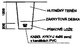
ŘEZ ULOŽENÍ V KRAJINCI KOMUNIKACE
