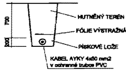
ŘEZ ULOŽENÍ NA p.p.č. 1998/4, 1998/3
