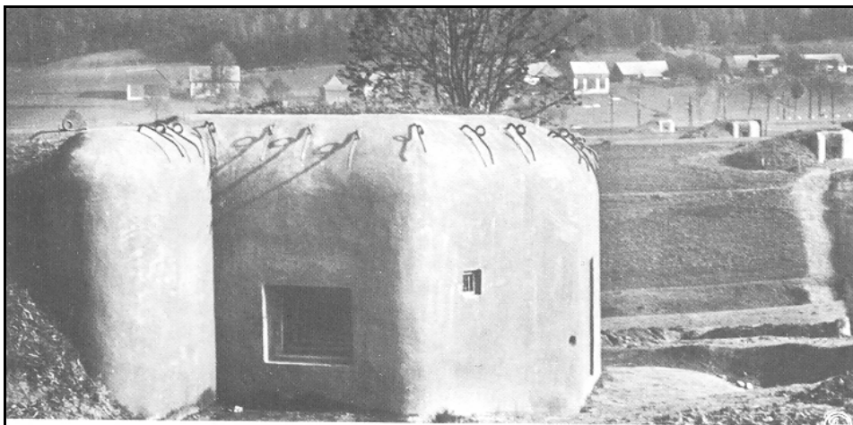
Nově postavené lehké opevnění – „ropík“ na úpatí Ovčí hory nad osadou Bedřichovka.
